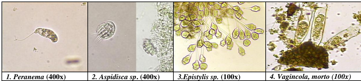
Figura 2 (2.1 – 2.4) Indicadores para a sobrecarga das estações de tipo aeração prolongada :
